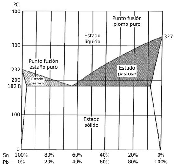
Figura 2: Temperatura de fusión de la aleación estaño-plomo.
